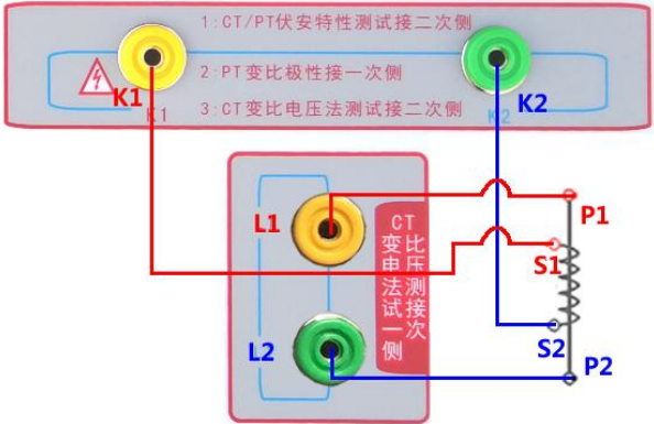
图 27 综合测试接线图
