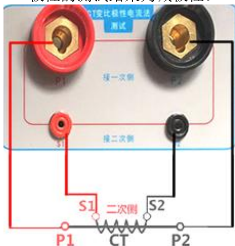
图 13，电流法 CT 变比极性 (角差比差) 接线图
