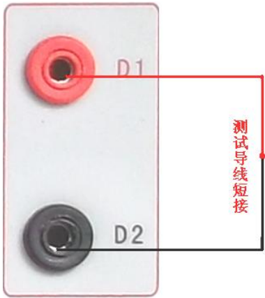
图 24，导线阻值清零接线图
